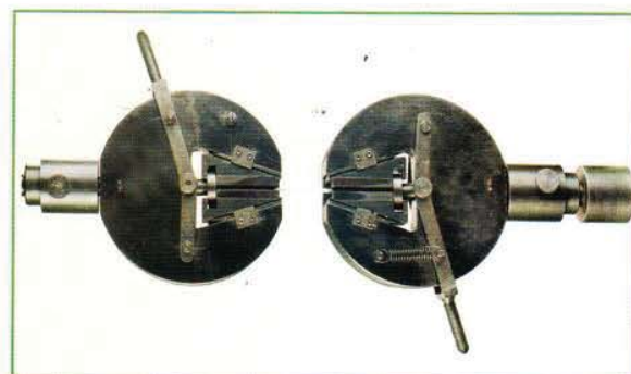
Wedge Type Grip
