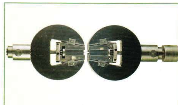
Vice cum Wedge Type Grip
